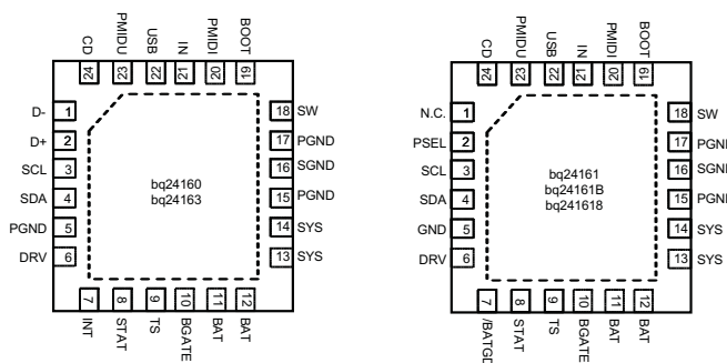
VQFN 24 Pins Top View
